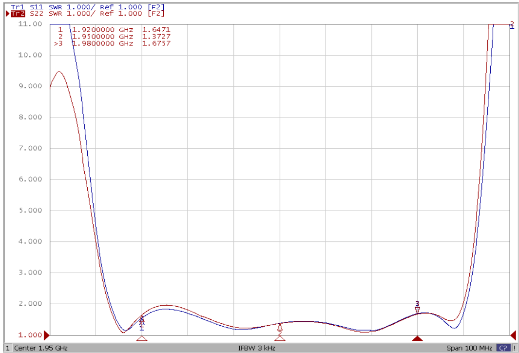
VSWR
